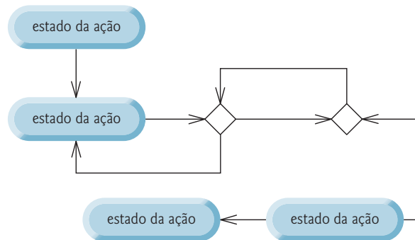
Figura 5.26 | Diagrama de atividade “não estruturado”.
