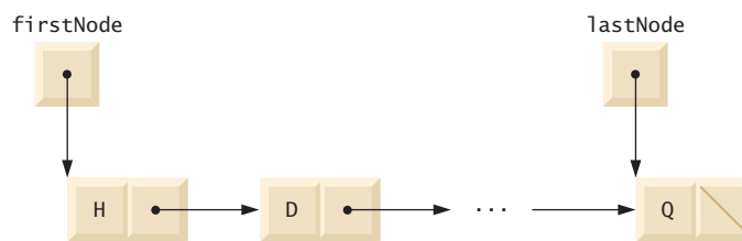
Figura 21.2 | Representação gráfica de lista encadeada.
