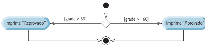
Figura 4.3 | Diagrama UML de atividades de instrução de seleção dupla if...else .
