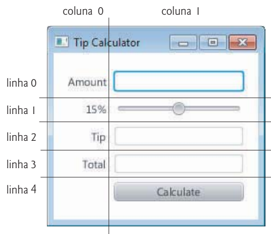
Figura 25.10 | GridPane da GUI Tip Calculator rotulado por suas linhas e colunas.
