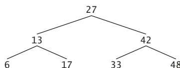
Figura 21.19 | A árvore de pesquisa binária com sete valores.
