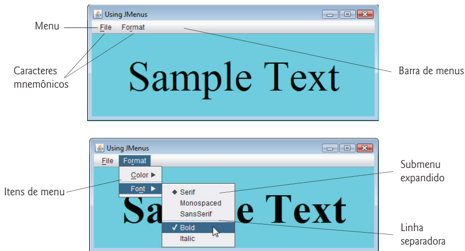
Figura 22.6 | Classe de teste para o MenuFrame.
