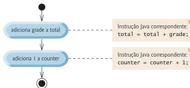
Figura 4.1 | Diagrama de atividades da estrutura de sequência.
