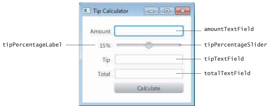
Figura 25.11 | Controles programaticamente manipulados do Tip Calculator rotulados com suas fx:ids .
