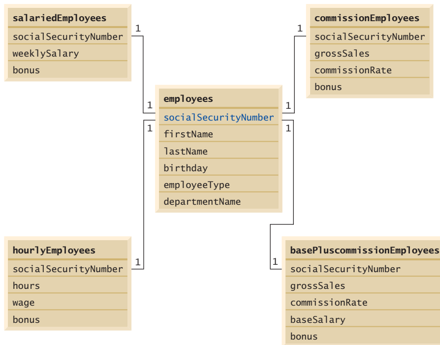
Figura 24.33 | Relacionamentos de tabela no banco de dados employees .
