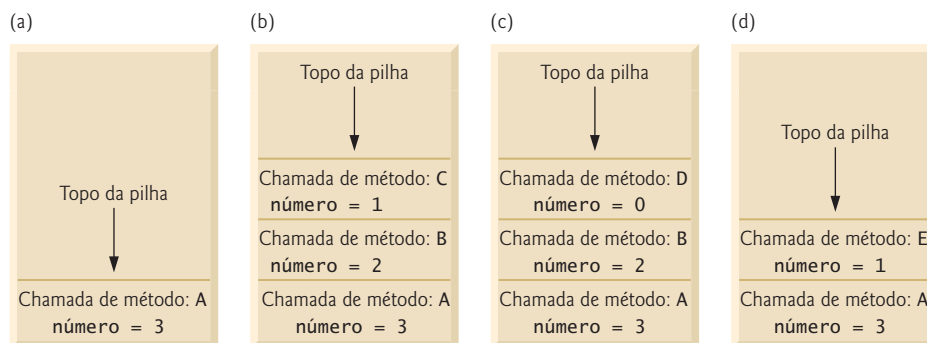
Figura 18.8 | Chamadas de método na pilha de execução do programa.
