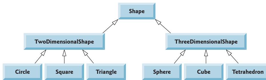
Figura 9.3 | Diagrama de classes UML da hierarquia de herança para Shapes.
