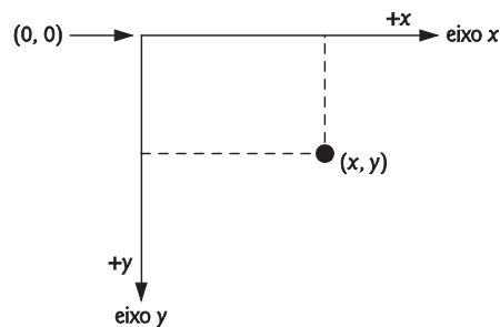
Figura 13.2 | Sistema de coordenadas Java. As unidades são medidas em pixels.
