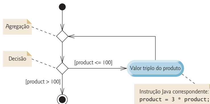
Figura 4.6 | Diagrama UML de atividades da instrução de repetição do... while .
