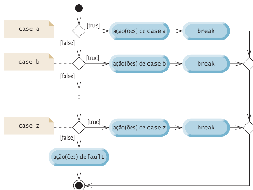
Figura 5.10 | Diagrama de atividades UML de instrução de seleção múltipla switch com instruções break .
