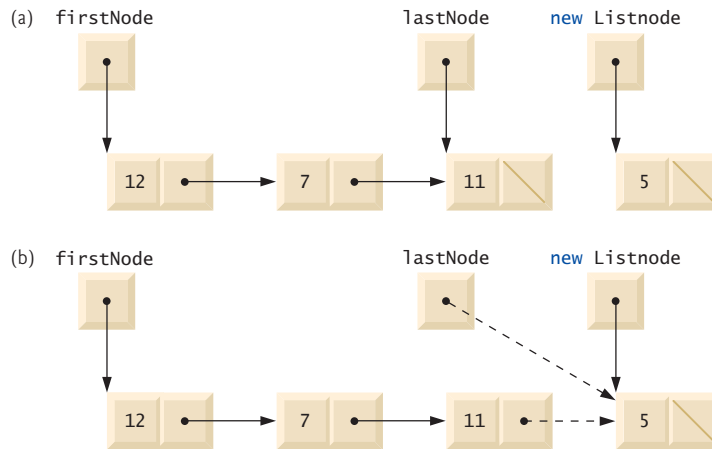
Figura 21.7 | Representação gráfica da operação insertAtBack .
