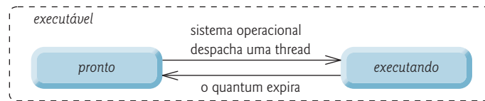
Figura 23.2 | Visualização interna do sistema operacional do estado executável do Java.
