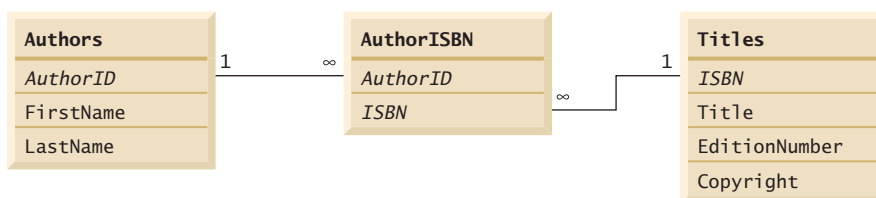
Figura 24.9 | Relacionamentos de tabela no banco de dados books.
