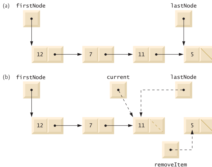
Figura 21.9 | Representação gráfica da operação removeFromBack .
