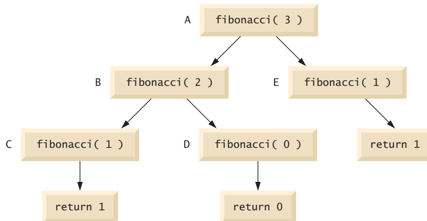
Figura 18.7 | Chamadas de método feitas dentro da chamada fibonacci(3) .
