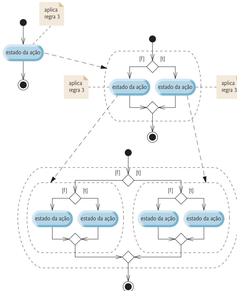
Figura 5.25 | Aplicando repetidamente a regra 3 da Figura 5.22 ao diagrama mais simples.
