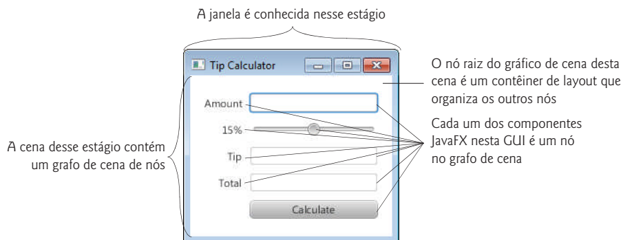
Figura 25.1 | Partes de uma janela de aplicativo JavaFX.
