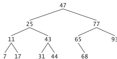
Figura 21.16 | Árvore de pesquisa binária contendo 12 valores.
