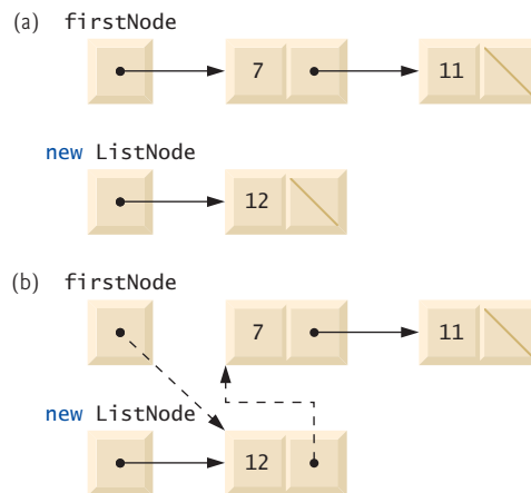
Figura 21.6 | Representação gráfica da operação insertAtFront .
