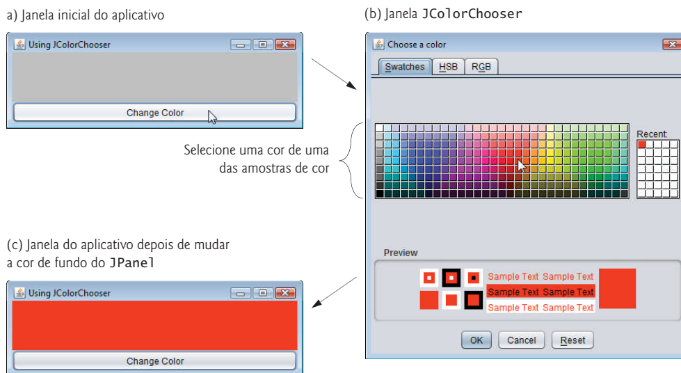
Figura 13.8 | Escolhendo cores com JColorChooser.
