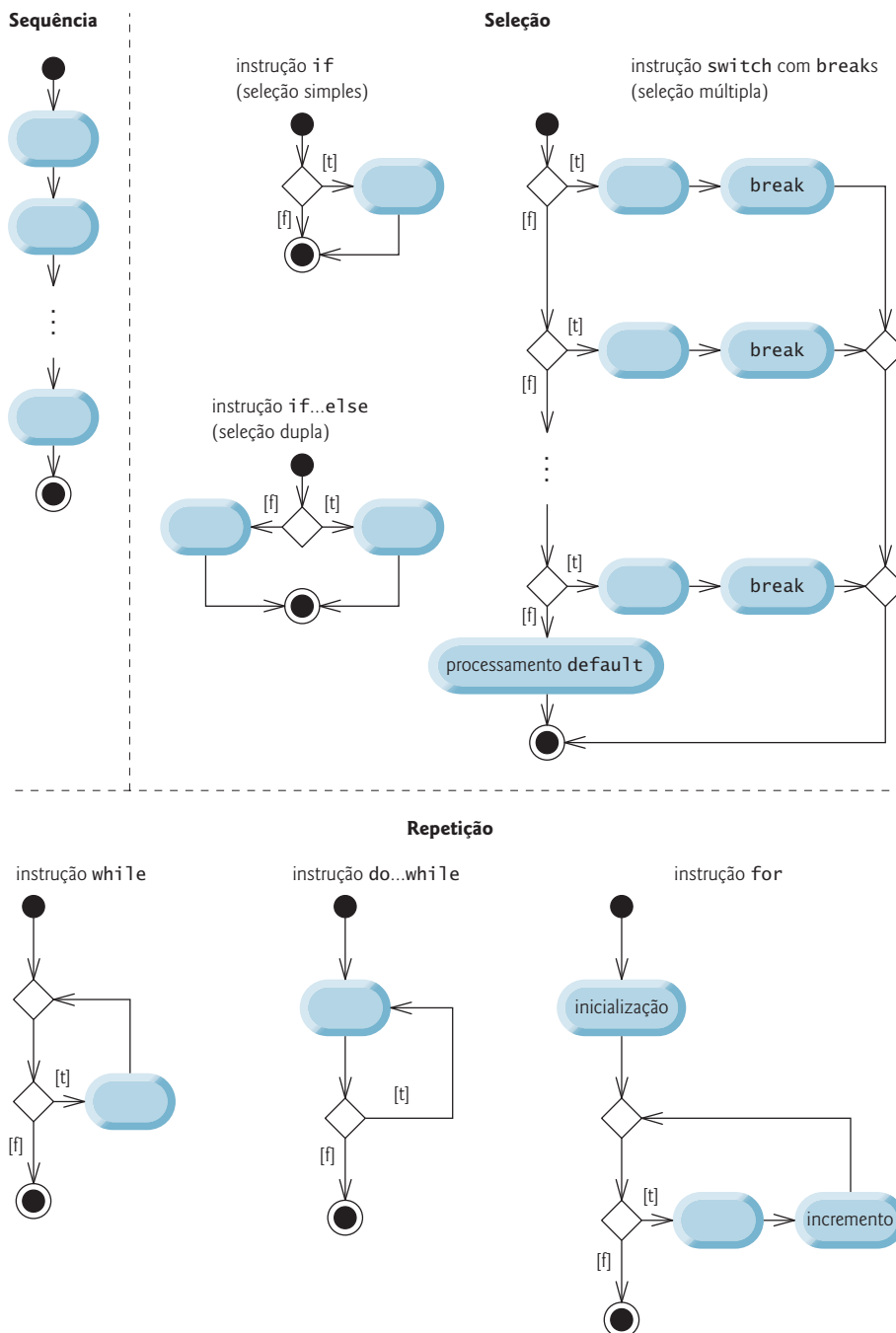
Figura 5.21 | As instruções de sequência de entrada única/saída única, seleção e repetição do Java.
