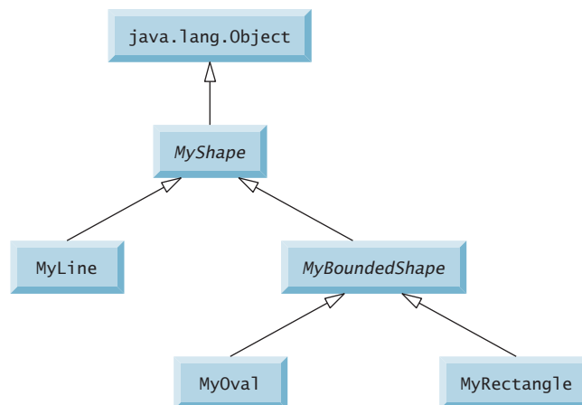
Figura 10.18 | A hierarquia MyShape com MyBoundedShape .
