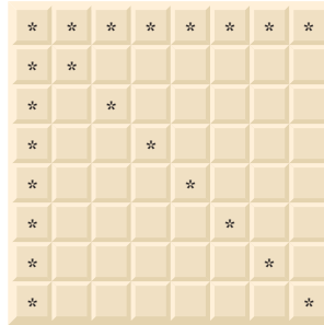
Figura 7.31 | Os 22 quadrados eliminados posicionando uma rainha no canto esquerdo superior.
