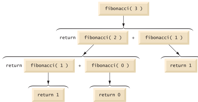
Figura 18.6 | Conjunto de chamadas recursivas para fibonacci(3) .
