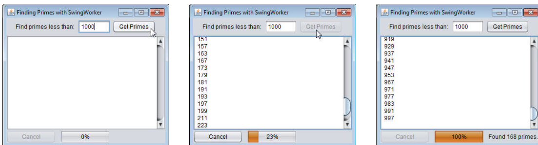
Figura 23.27 | Usando um SwingWorker para exibir números primos e atualizar uma JProgressBar enquanto os números primos são calculados.
