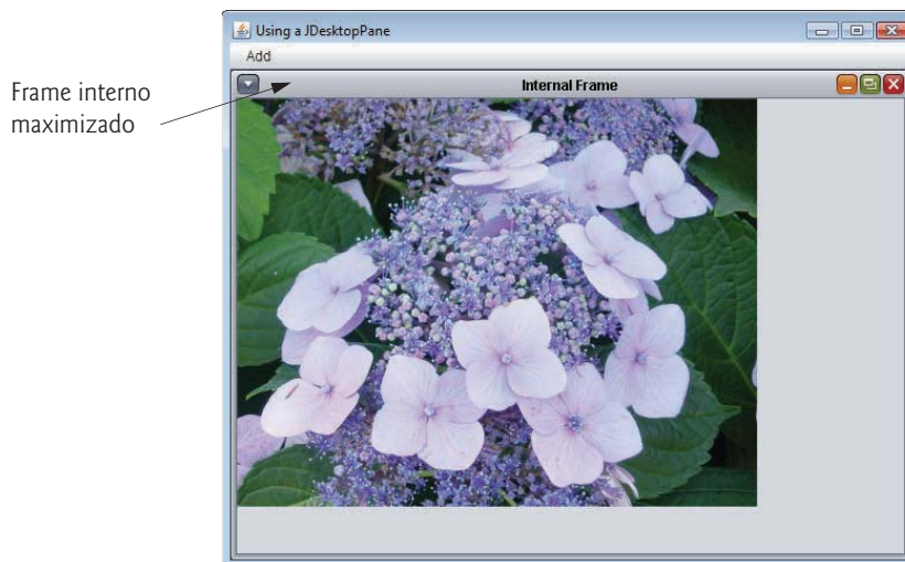
Figura 22.12 | Classe de teste para o DesktopFrame.
