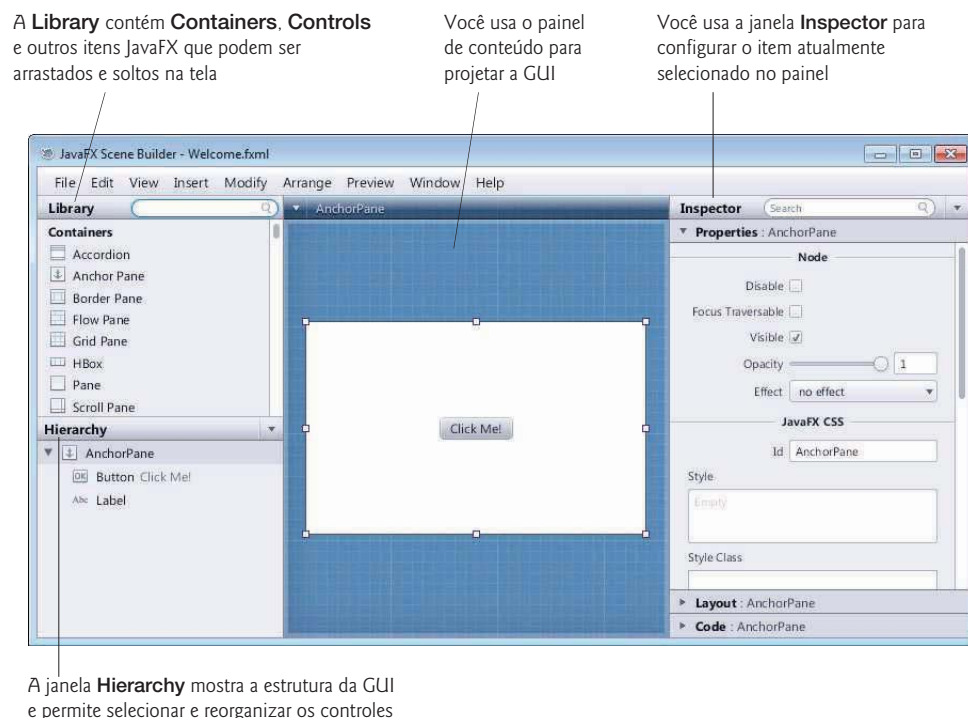
Figura 25.7 | O JavaFX Scene Builder exibindo a GUI padrão em Welcome.fxml .
