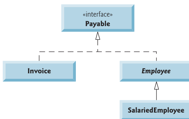
Figura 10.10 | Diagrama de classes da UML da hierarquia da interface Payable .
