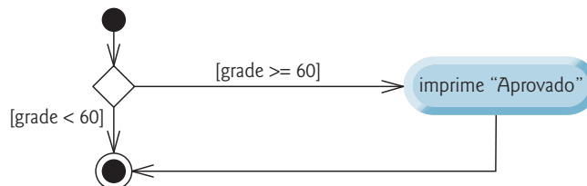
Figura 4.2 | Diagrama UML de atividades de uma instrução de seleção única if .
