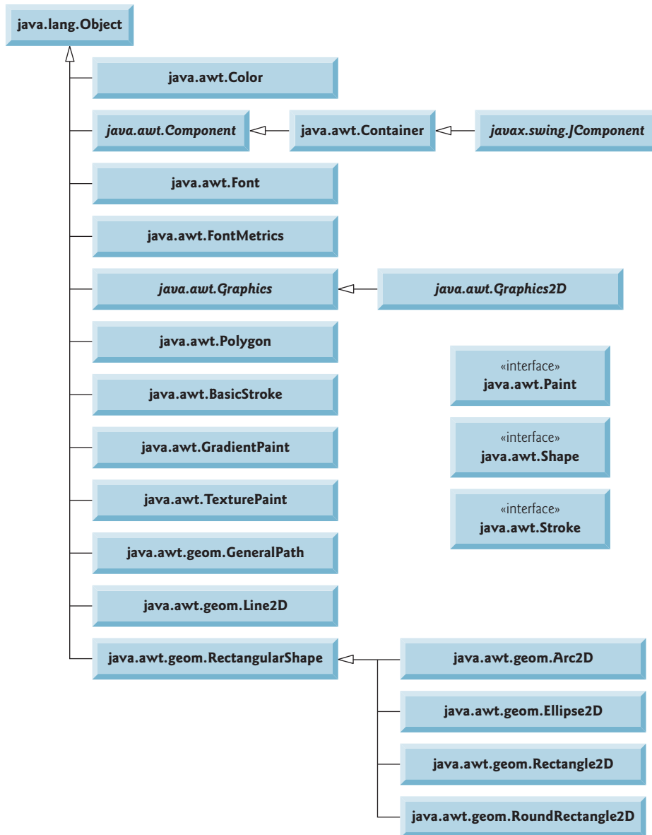
Figura 13.1 | As classes e interfaces utilizadas neste capítulo são provenientes das capacidades gráficas originais do Java e da Java 2D API.
