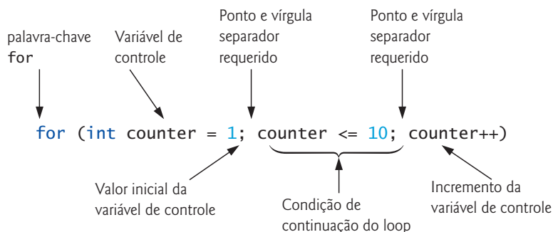
Figura 5.3 | Componentes de cabeçalho de instrução for .
