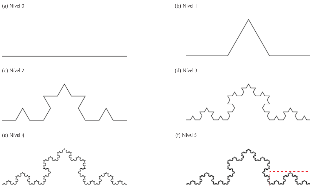
Figura 18.12 | Fractal da Curva de Koch.
