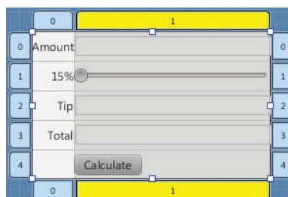
Figura 25.14 | GridPane com colunas dimensionadas para ajustar-se ao conteúdo.
