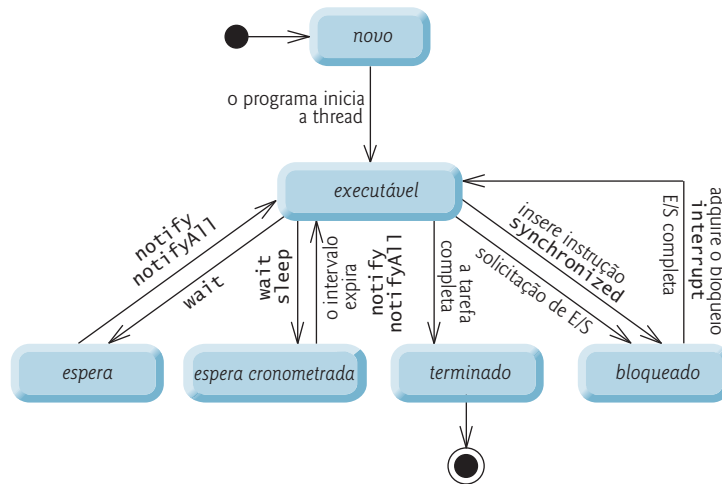
Figura 23.1 | Diagrama de estado de ciclo de vida da thread.
