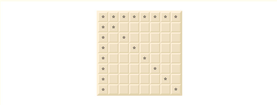
Figura 18.20 | Os quadrados eliminados pela colocação de uma rainha no canto superior esquerdo de um tabuleiro.
