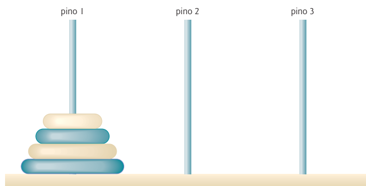
Figura 18.10 | As Torres de Hanói para o caso com quatro discos.
