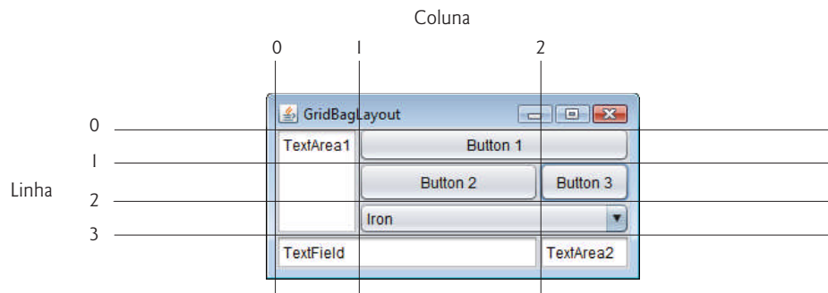
Figura 22.18 | Projetando uma GUI que utilizará GridBagLayout .
