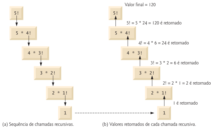
Figura 18.2 | Avaliação recursiva de 5! .
