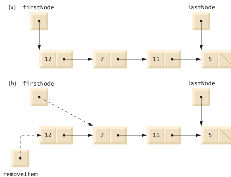
Figura 21.8 | Representação gráfica da operação removeFromFront .
