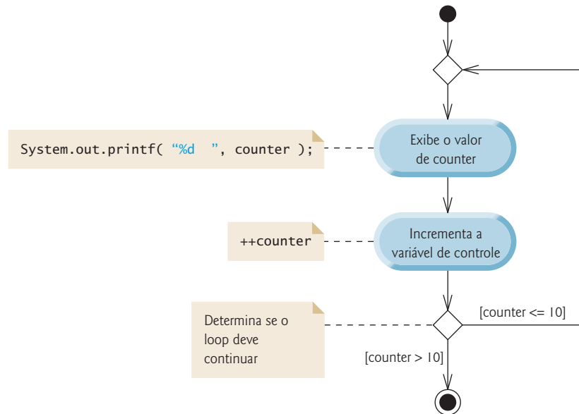
Figura 5.8 | Diagrama de atividades UML para a instrução de repetição do...while .
