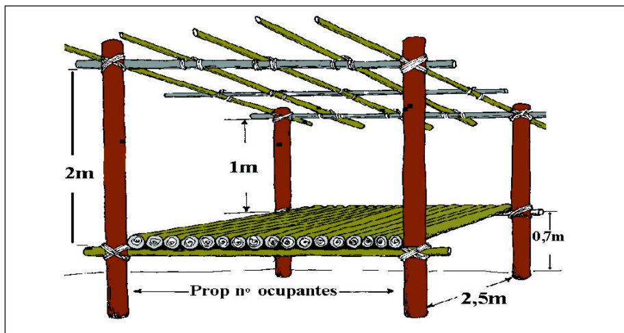
Fig 5-17. Tapiri simples (medidas)
