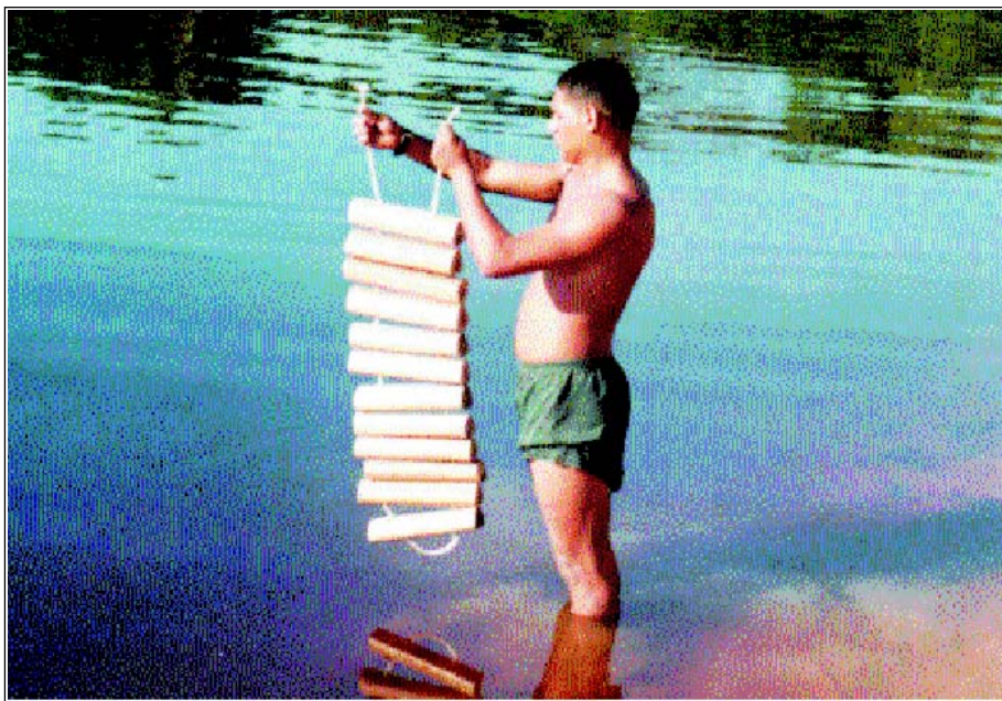
Fig 4-24. Bóia de talo de buriti (pronta para ser utilizada)
