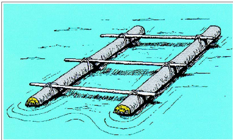
Fig 4-35. Tipo de jangada (detalhes da montagem)
