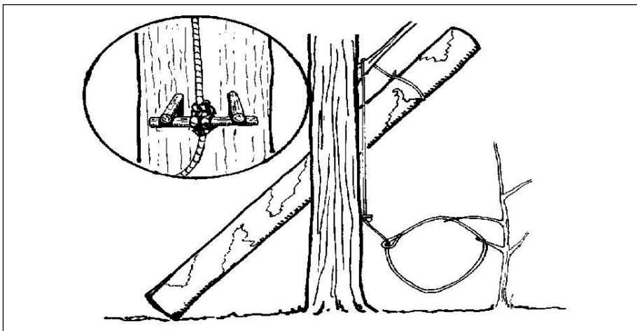
Fig 6-39. Mundéu associado a laço
