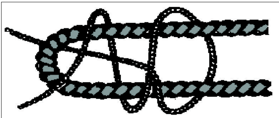
Fig 4-17. Nós de escota (para cordas de diâmetro diferentes)
