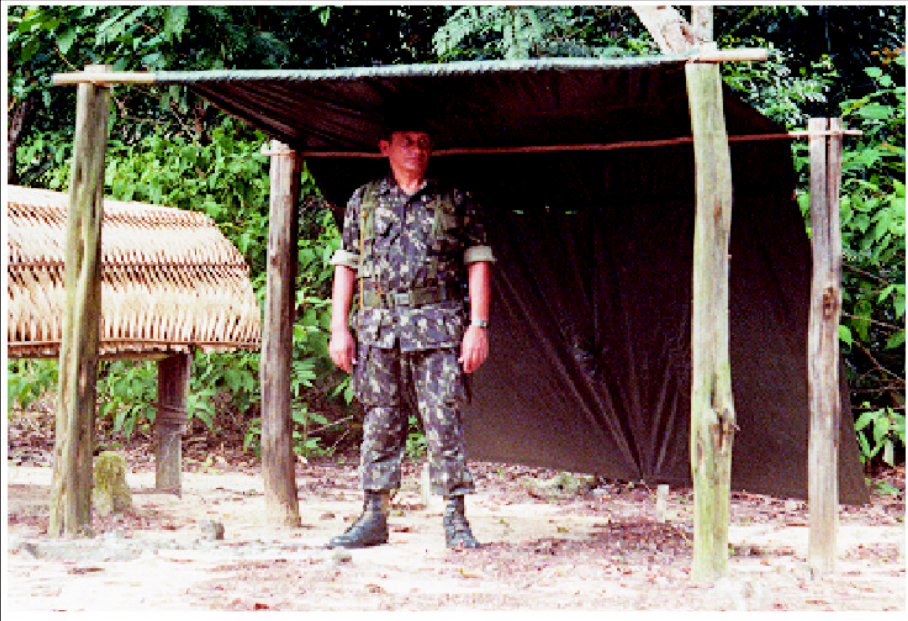
Fig 5-13. Abrigo improvisado utilizando dois ponchos presos em estacas e suspensos do solo
