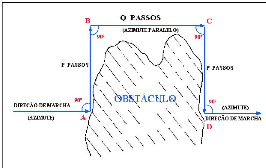
Fig 4-9. Desvio de um obstáculo pelo processo da compensação com passos e ângulos retos
