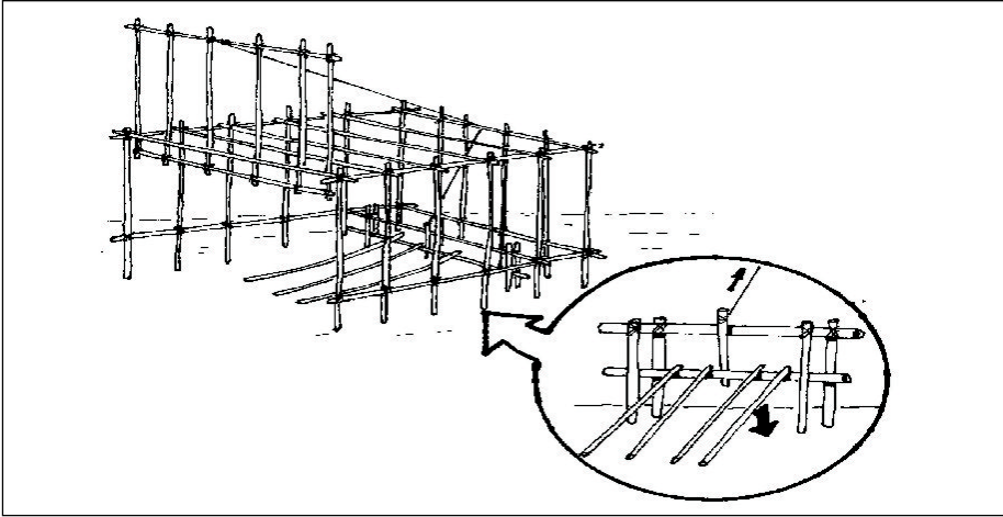
Fig 6-37. Chiqueiro (Obs: para manter qualquer felino no seu interior os troncos deverão estar unidos uns aos outros, assim a armadilha terá firmeza e solidez)
