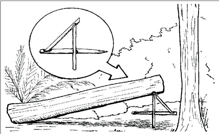
Fig 6-38. Mundéu
