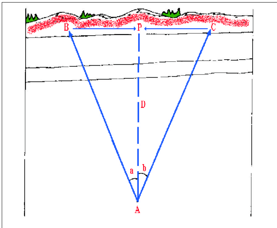
Fig 4-7. "Off-Set" (a ou b, ângulo somado ou subtraído do azimute da direção AP)
