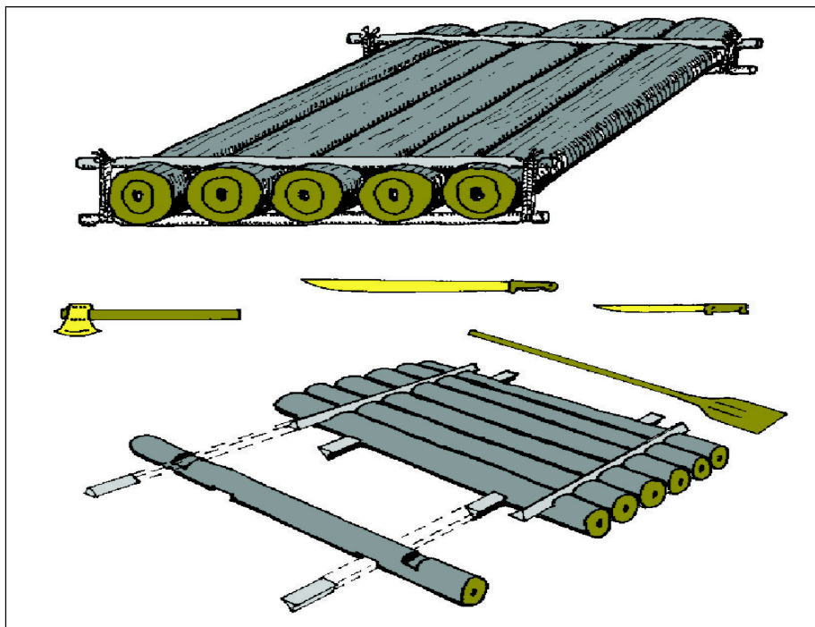
Fig 4-34. Jangada (apenas para mostrar a construção; necessitará de mais troncos transversais)
